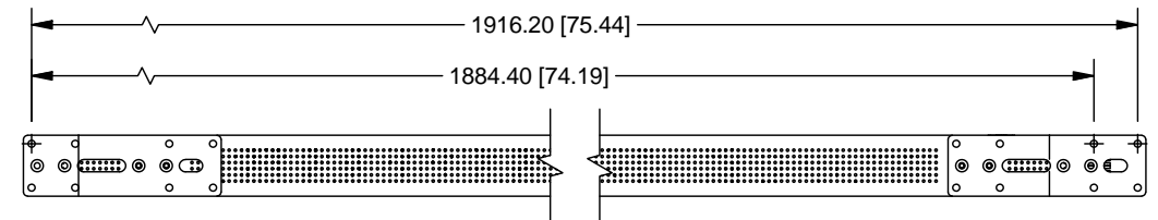
OPTION D - MB-0005-IPT7
