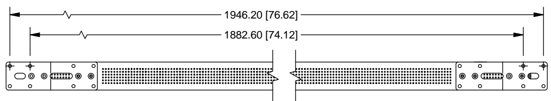
OPTION C - MB-0005-IPT7
